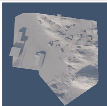
Sol skygge analyse 21 Mars kl.15
